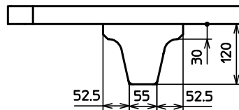
断面A-A
