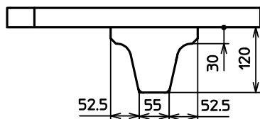
断面A-A
