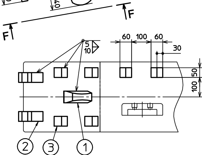
F矢視図
