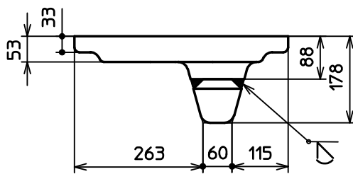
断面A-A
